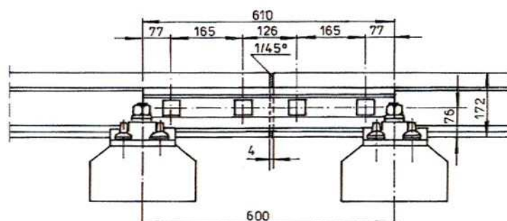
Rys. 3 Złącze szynowe izolowane klejono-sprężone z łóbkami czterootworowymi Rysunek górny: szyny 49E1, rysunek dolny szyny 60E1
