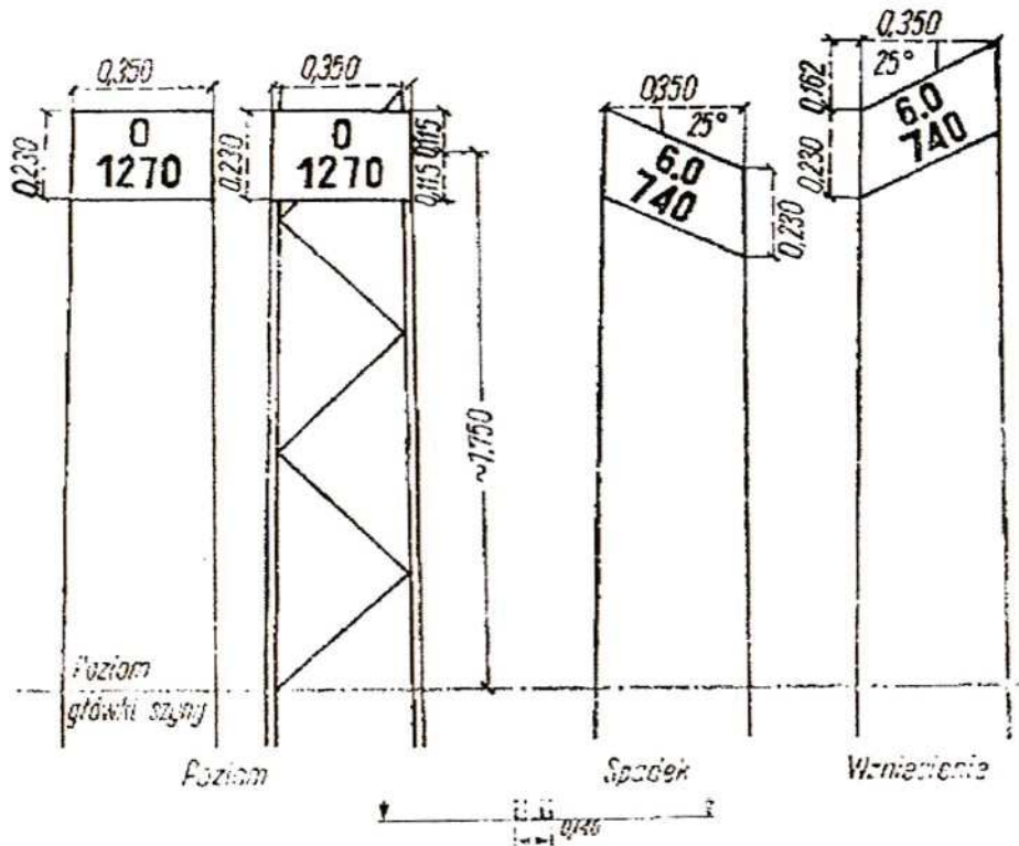
Rys.3 Znak pochylenia na liniach zelektryfikowanych
