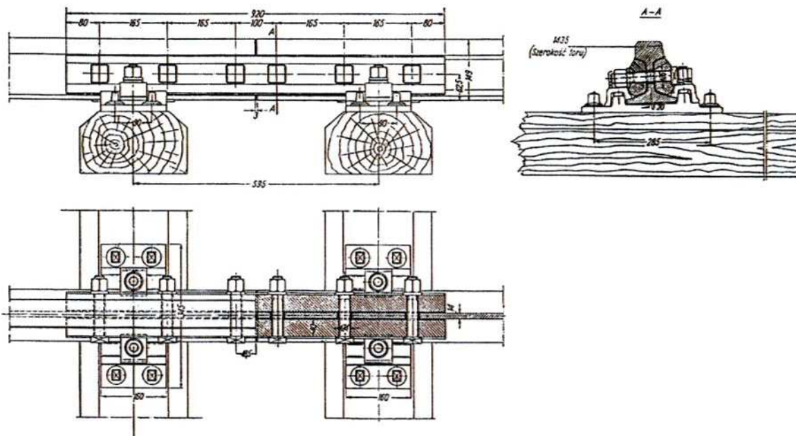
Rys. 3 Złącze szyn 49E1 wiszące
