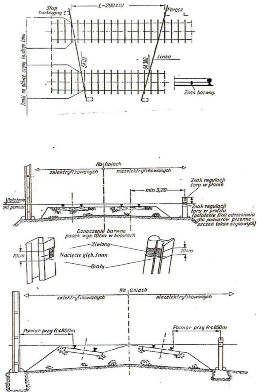
Rys.2 Zasady instalowania punktów stałych i dokonywania pomiarów
