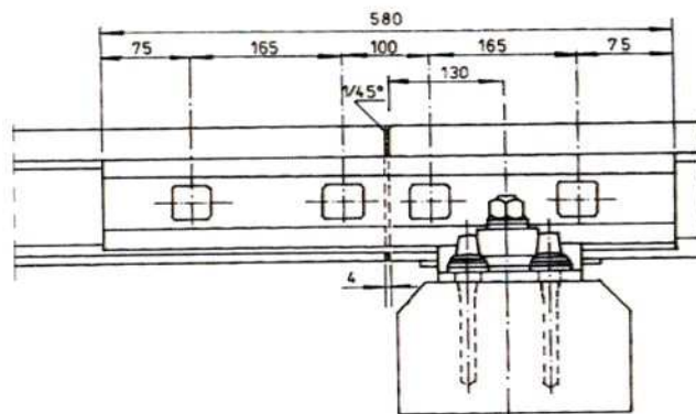
Rys. 4 Złącze szynowe izolowane klejono-sprężone z łubkami czterootworowymi z szyn 49E1.
