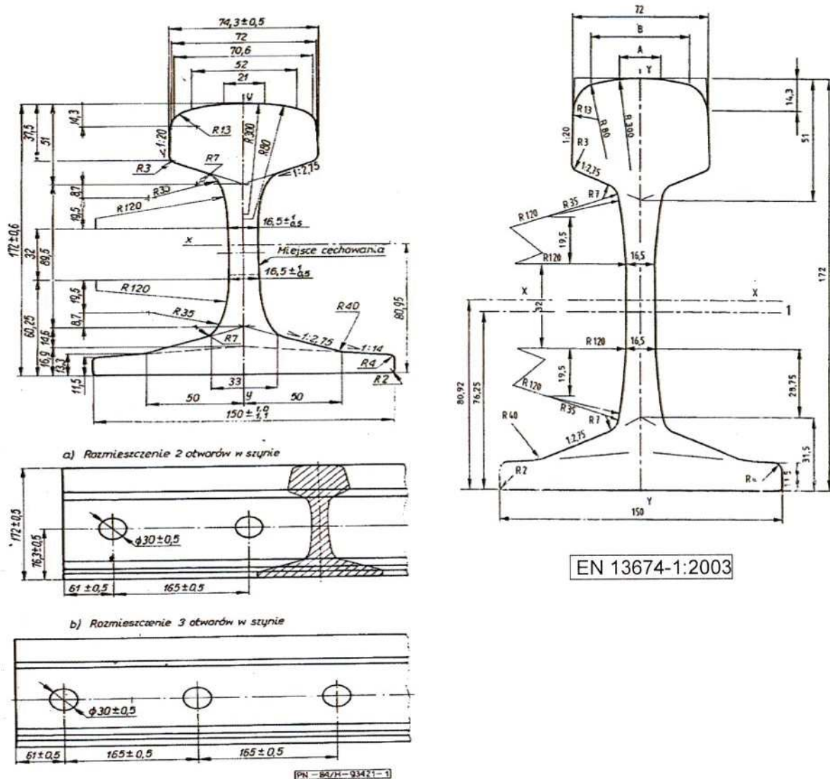
Rys. 1 Przekrój poprzeczny szyny 60E1
