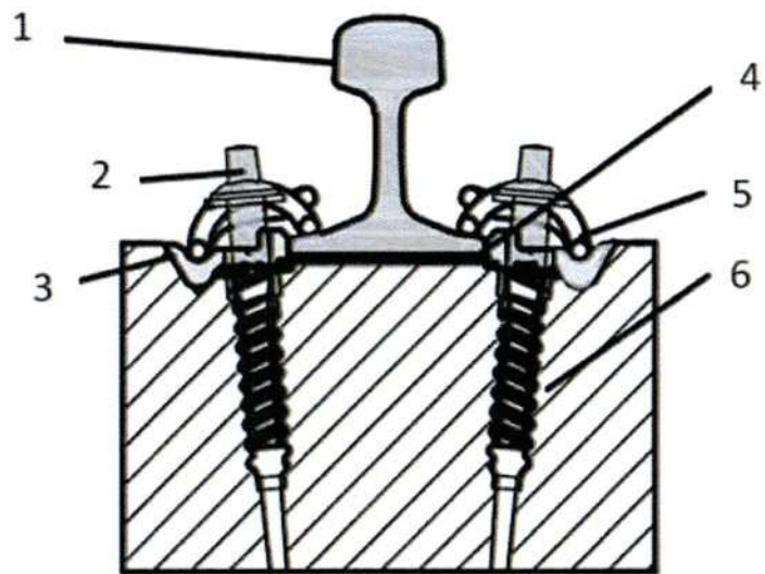
Rys. 3 Przytwierdzenie typu W-14 do podkładów strunobetonowych PS-94
