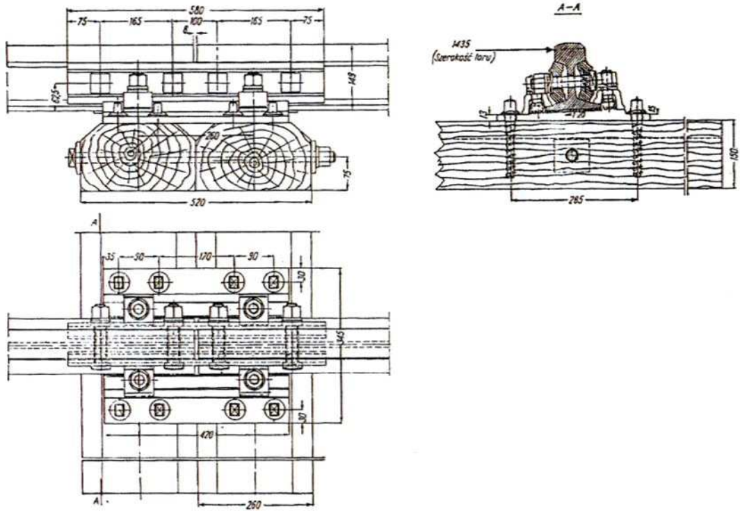
Rys. 4 Złącze szyn 49E1 podparte
