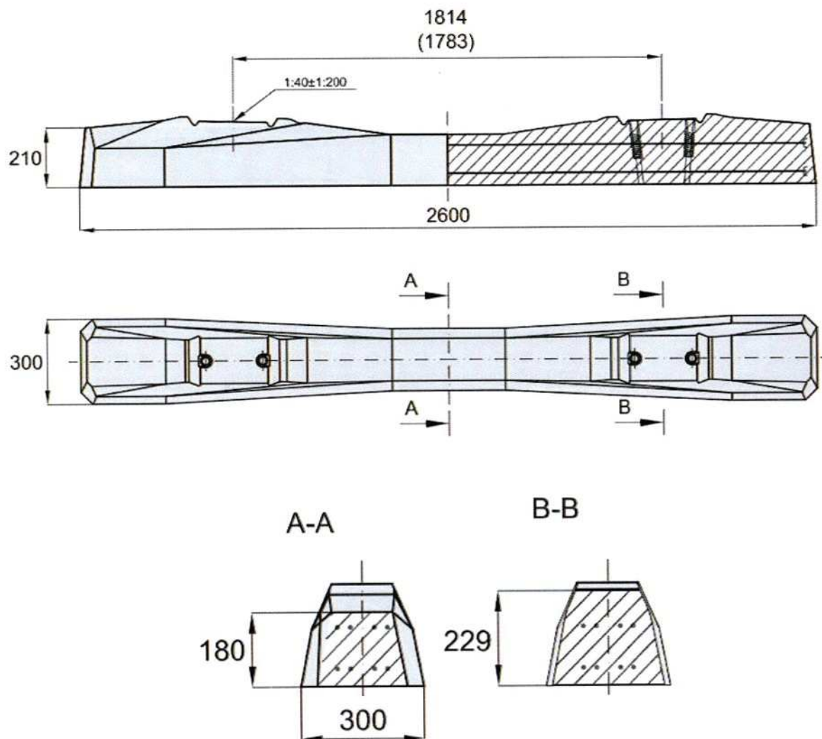
Rys. 3 Podkład strunobetonowy PS- 94 przystosowany do przytwierdzenia sprężystego W-14
