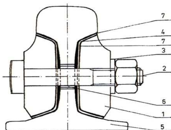
Rys.1 Elementy złącza szynowego izolowanego klejono-sprężonego
