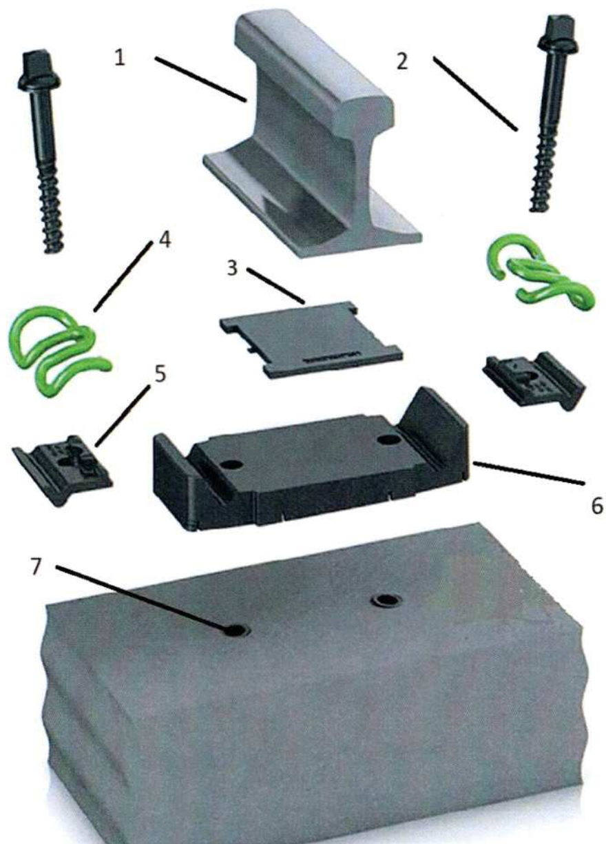
Rys. 4 Przytwierdzenie typu DFF 21 do podkładów betonowych
