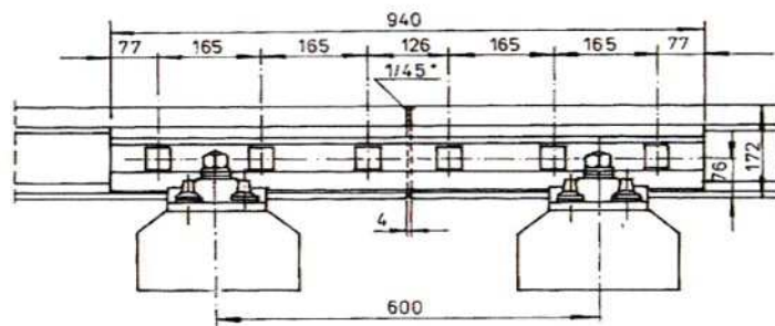
Rys. 2 Złącze szynowe izolowane klejono-sprężone z łóbkami sześciootworowymi Rysunek górny: szyny 49E1, rysunek dolny szyny 60E1
