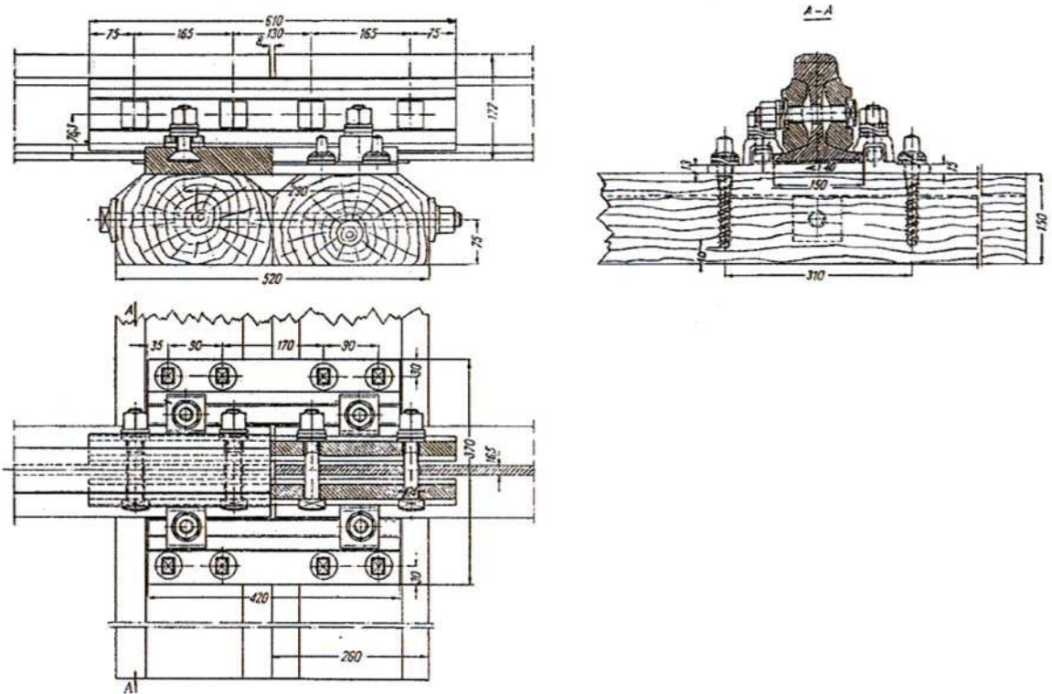
Rys. 2 Złącze szyn 60E1 podparte
