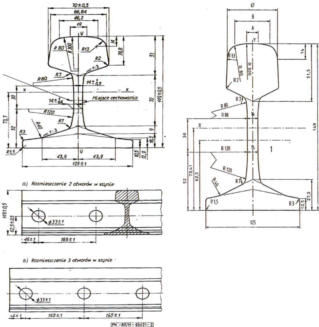
Rys. 2 Przekrój poprzeczny szyny 49E1
