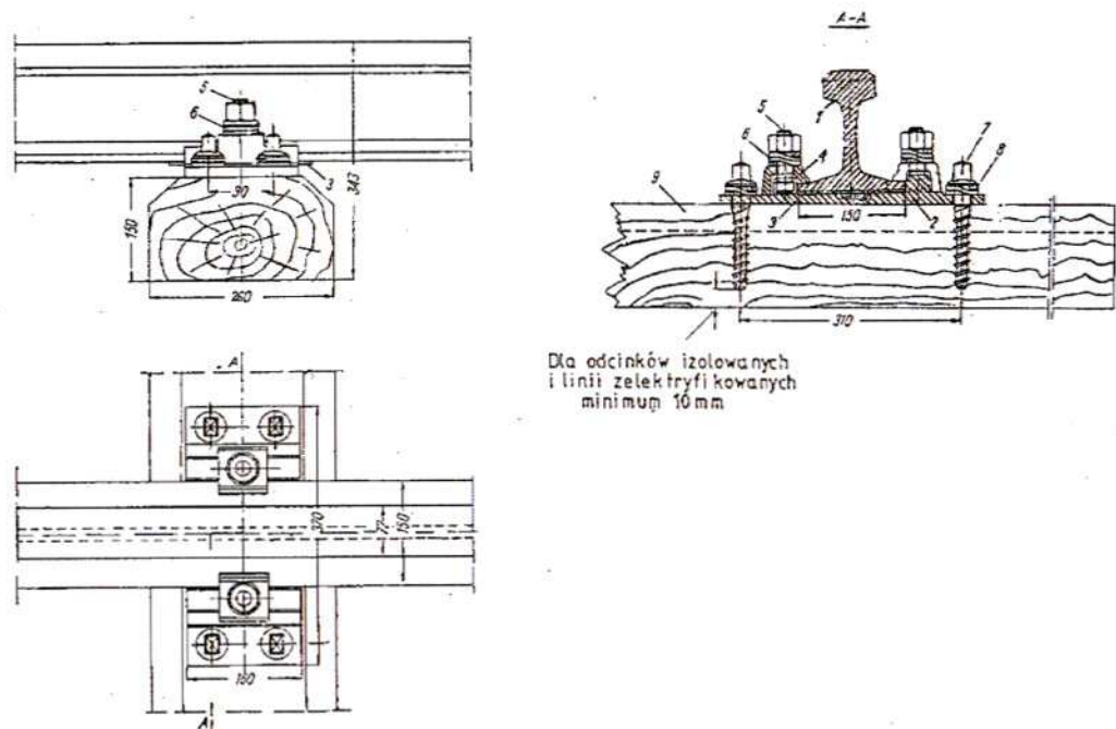
Rys.1 Przytwierdzenie typu K szyny UIC60(60E1) do podkładów drewnianych
