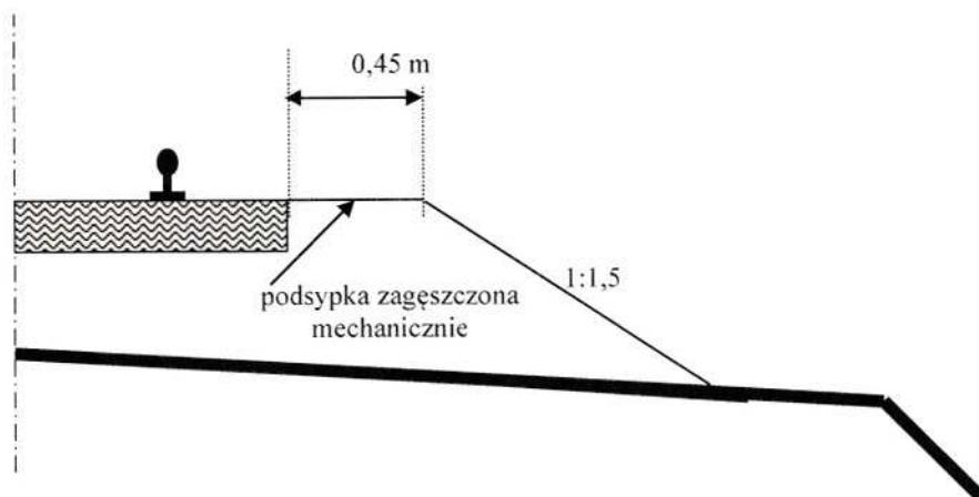
Rys. 3.1 Ukształtowanie przyzmy podsyпки w torze bezsypkowym.
