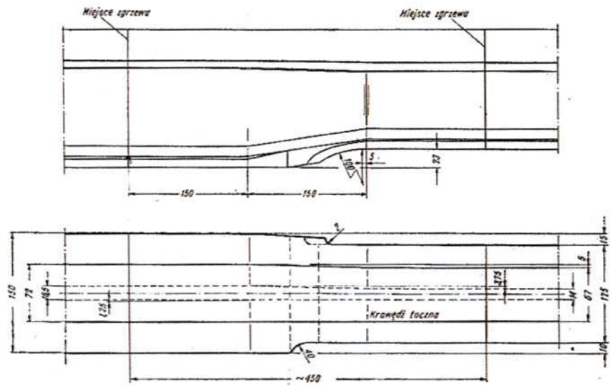
Rys. 4 Złącze szyn 49E1 podparte
