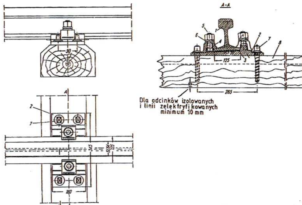
Rys.2 Przytwierdzenie typu K szyny S49(49E1) do podkładów drewnianych
